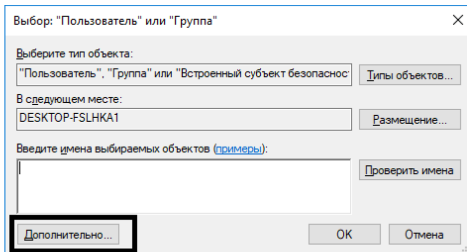
Рисунок 4.22 Окно Выбора
