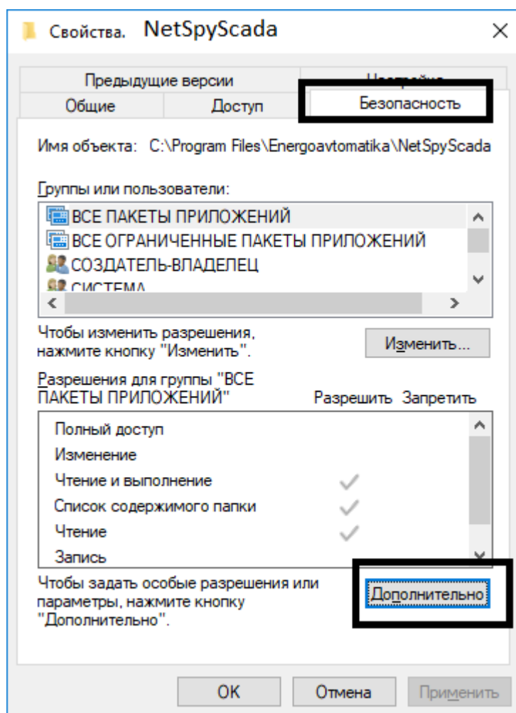
Рисунок 4.19 Свойства NetSpySKRScada
