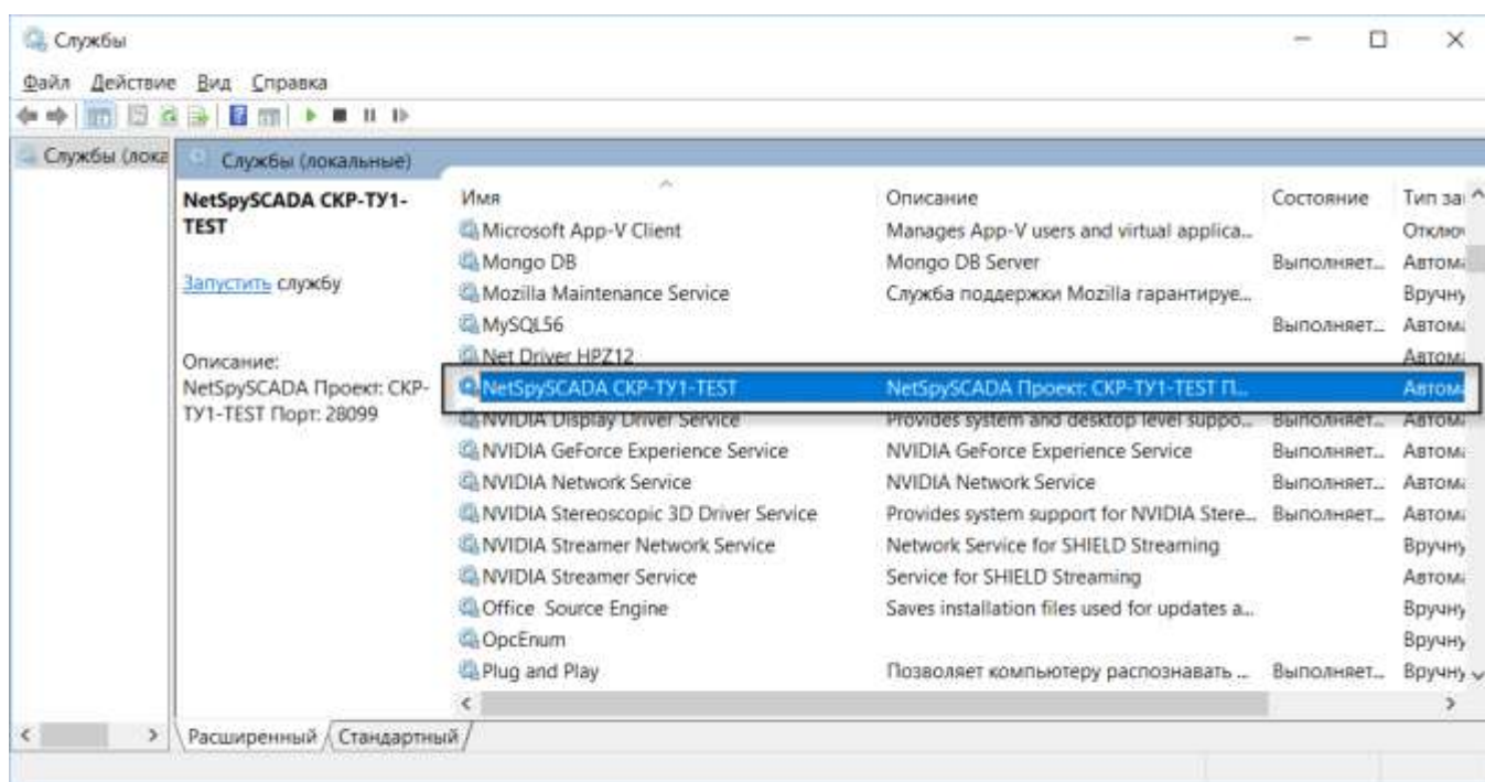
Рисунок 4.27 Окно служб
