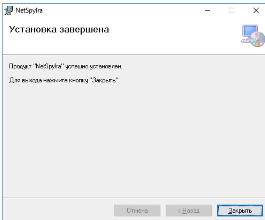
Рисунок 4.18 – Подтверждение установки
