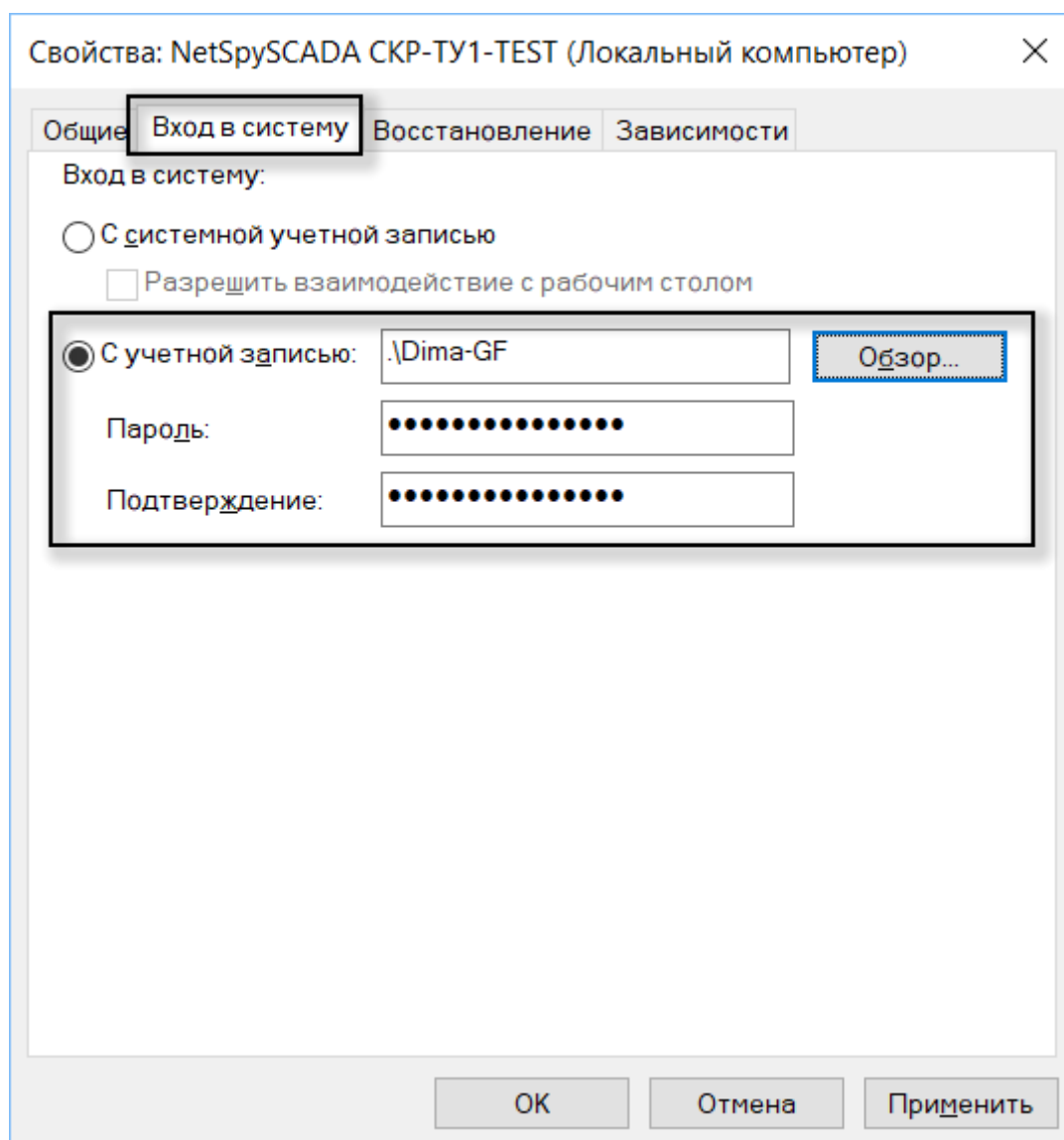
Рисунок 4.28 Окно свойств
